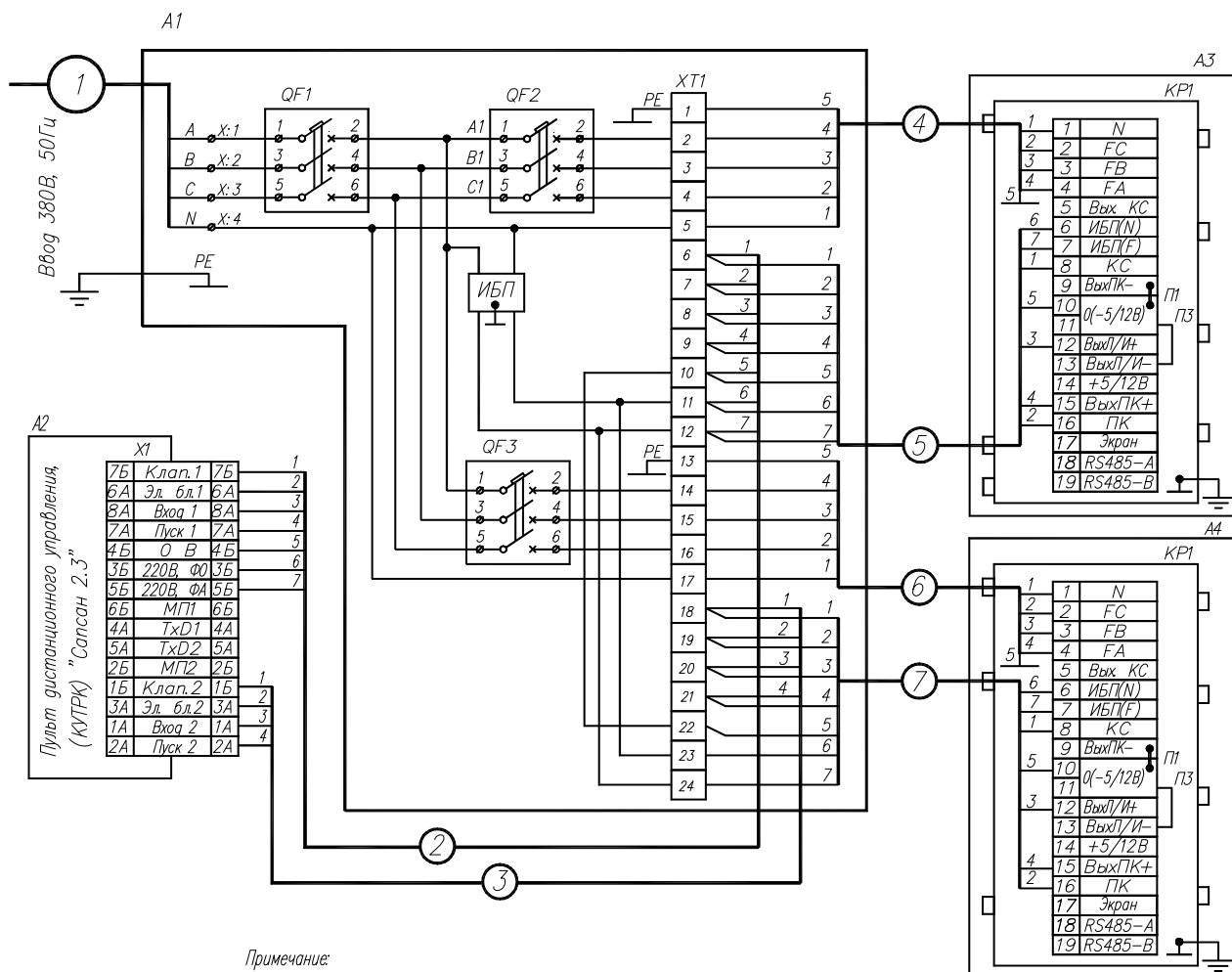
Рис. 5.1 Схема электрическая подключения ТРК (УТ) "Топаз-511" в дистанционном режиме с ПДУ, КУТРК "Солсан 2.3".
