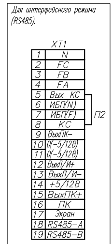
Рис. 6 Остальное по рис. 1 KP1
