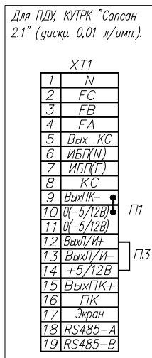
Рис. 4 Остальное по рис. 1 KP1
