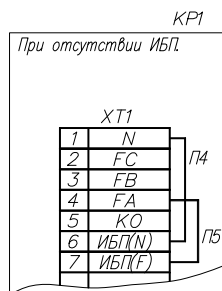
Рис. 7 Остальное по рис. 1-6.
