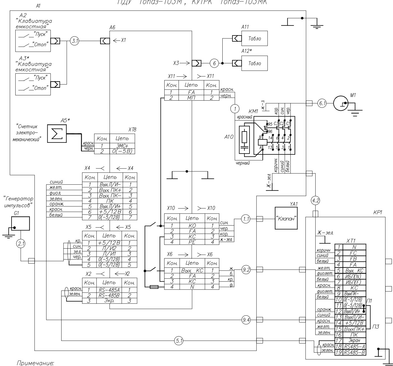
Рис. 1. ТРК (УТ) "Тоназ-511" для подключения к ПДУ "Тоназ-103М", КУТРК "Тоназ-103МК"
