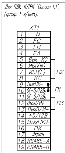
Рис. 2 Остальное по рис. 1 KP1
