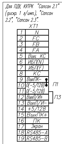
Рис. 3 Остальное по рис. 1 KP1
