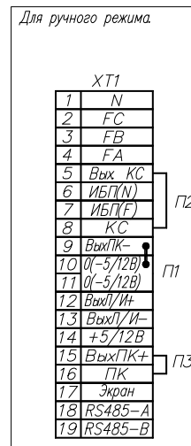
Рис. 5 Остальное по рис. 1 KP1
