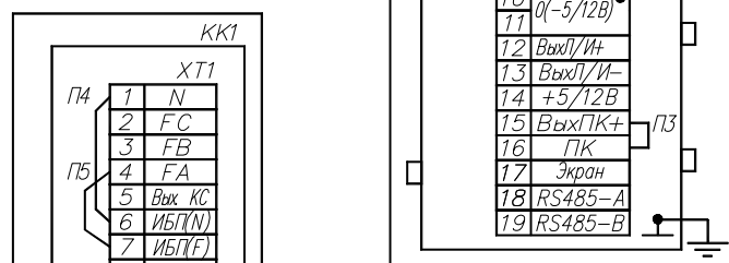
Рис. 4.2 Схема установки перемычек при отсутствии ИБП. Остальное по рис. 4.1.
