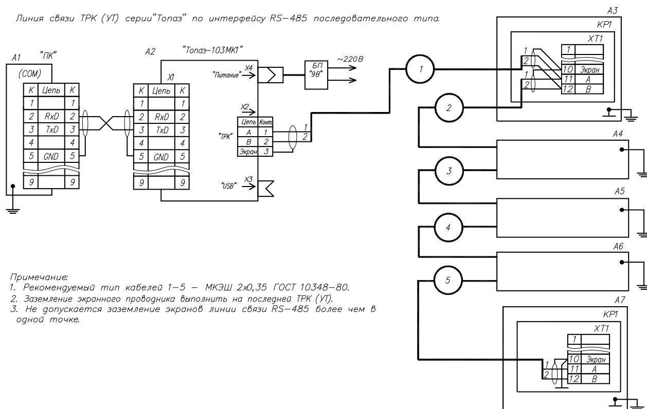
Рисунок Е.2 Линия связи "RS-485" для АЗС с ТРК "ТОПАЗ"
