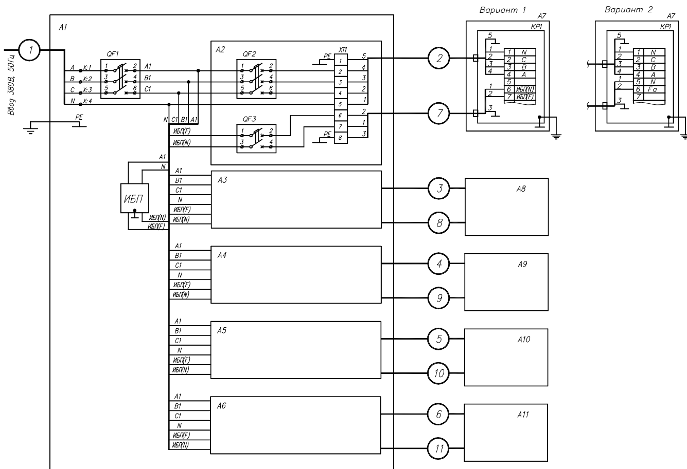
Рис. 1.1 Схема электрическая подключения силовой части ТРК (УТ) "Топаз" со всасывающей гидравликой. (Схема коробки распределительной KP1 по варианту 1, 2 соответствует схеме электрической соединений ТРК)
