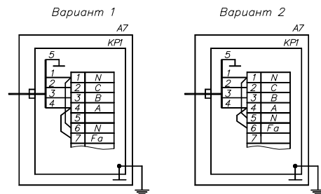
Рис. 1.2 Подключение ТРК (УТ) "Топаз" при отсутствии ИБП с разными вариантами исполнения KP1. Остальное по рис. 1.1.
