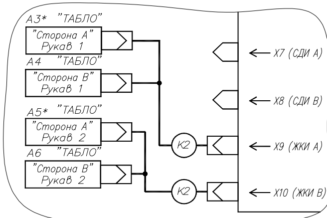
Рис. 1.3 Остальное по Рис. 1.1
