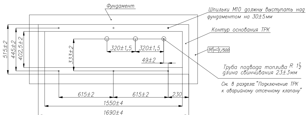
Рисунок А.2 ТРК "Топаз-230-2Х-Х000/00 К"
