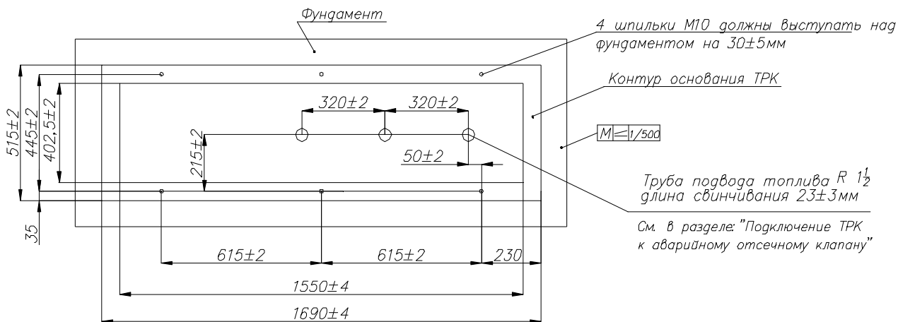
Рисунок А.1 ТРК "Топаз-230-2Х-Х000/00"
