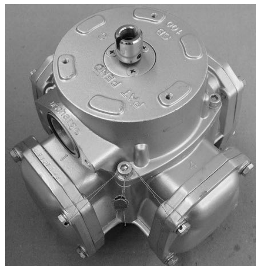
Рисунок Г.3 Пломбировка измерителя объёма
