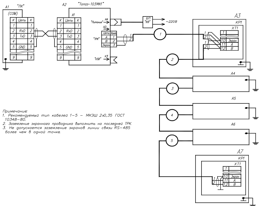
Рисунок Д.2 Линия связи "RS-485" для АЗС с ТРК "ТОПАЗ"
