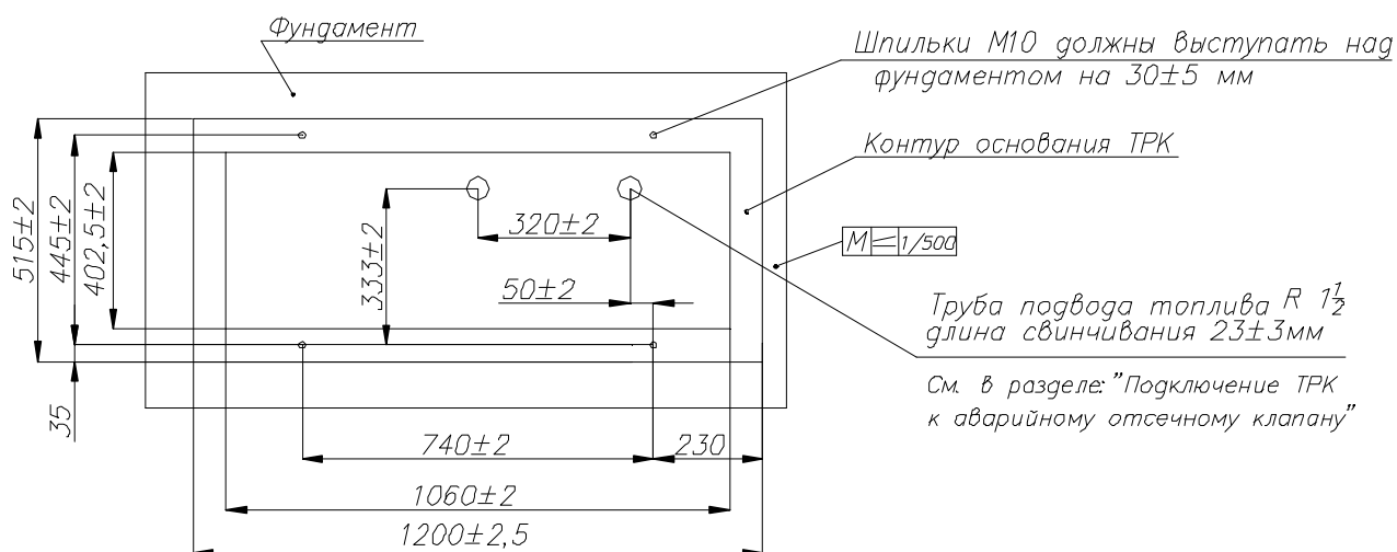
Рисунок А.2 ТРК "Топаз-220-2Х-Х000/00 К"
