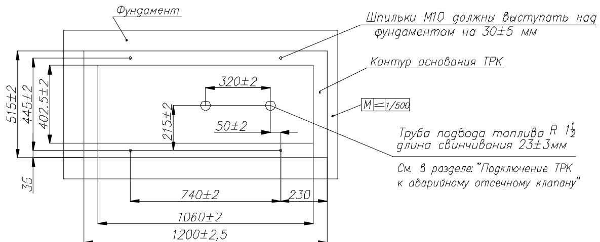
Рисунок А.1 ТРК "Топаз-220-2X-X000/00"
