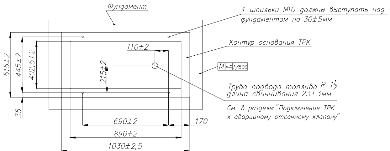
Рисунок А.1 ТРК "Топаз-210-2X-X000/00"
