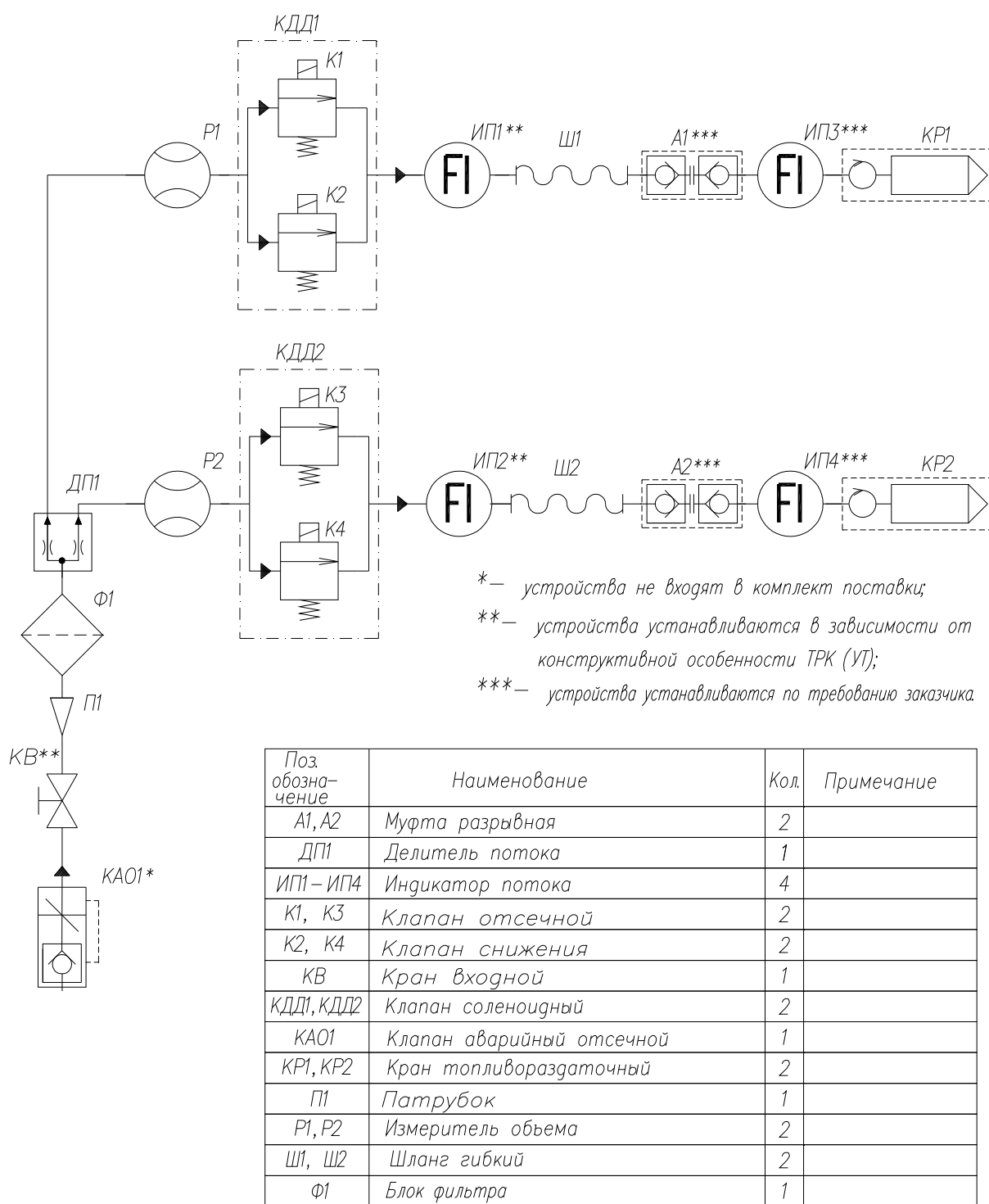
Рисунок Ж.1 Схема гидравлическая принципиальная гидравлической линии ТРК. Количество гидравлических линий в ТРК - 1 шт.
