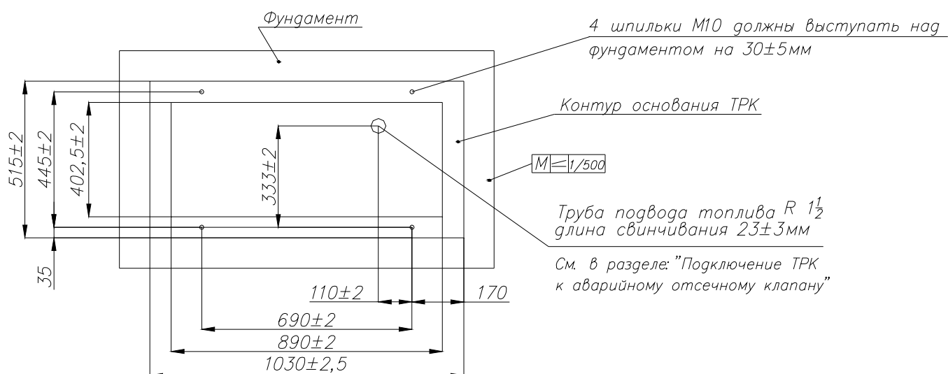
Рисунок А.2 ТРК "Топаз-210-2Х-Х000/00 К"
