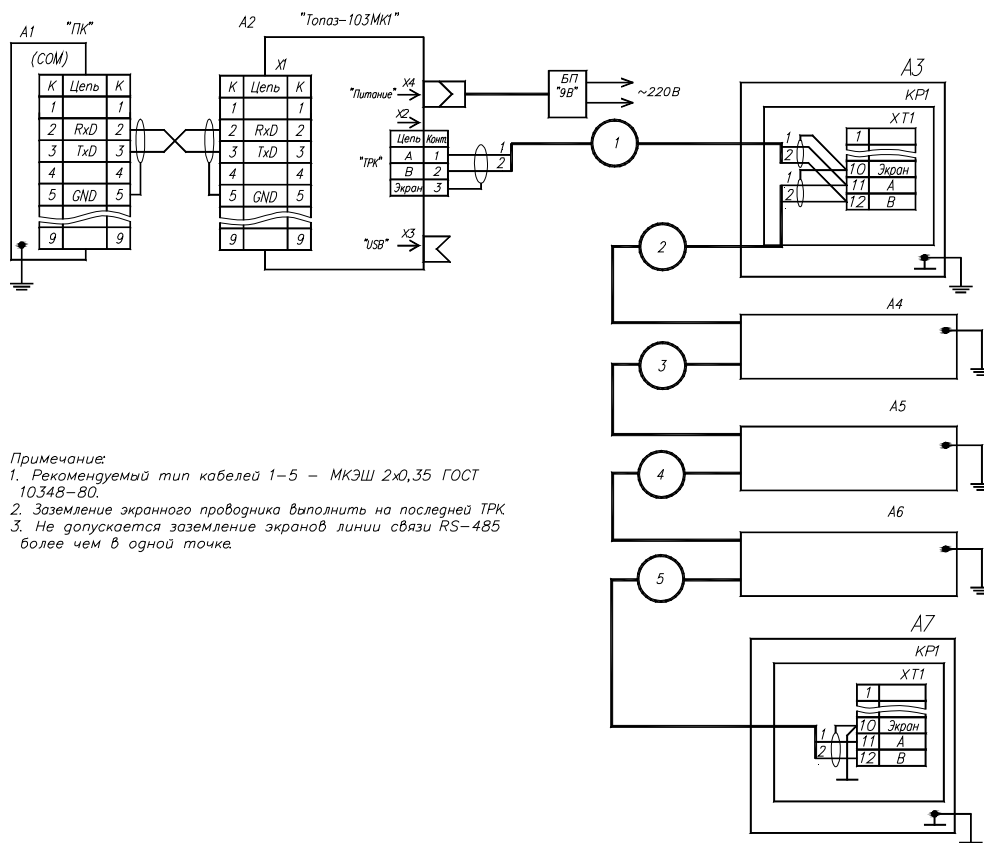
Рисунок Е.2 Линия связи "RS-485" для АЗС с ТРК "ТОПАЗ"
