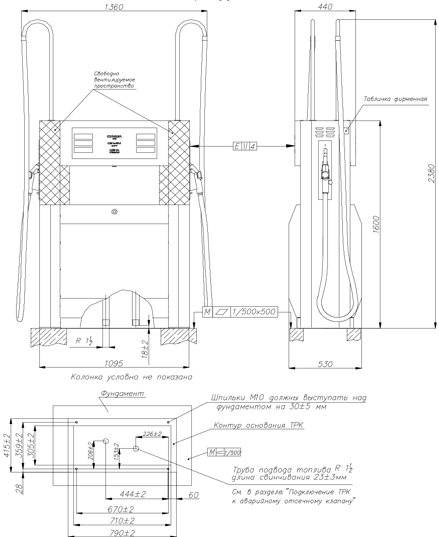
Рисунок А.1 Колонка топливораздаточная "Топаз-420-XX-X000/00"
